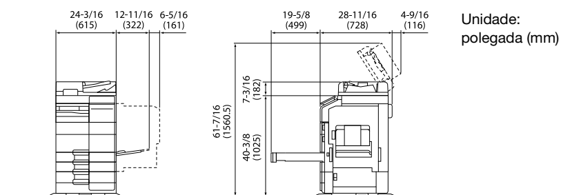
Unidade principal + DK-705 + PC-216
