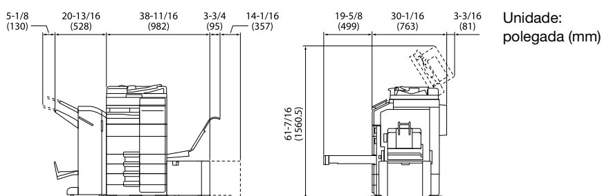
Unidade principal + DK-705 + FS-539 SD + PC-216 + LU-302 + MK-730 + CU-102
